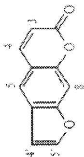
Psoralen
