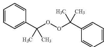
Dicumyl peroxide
